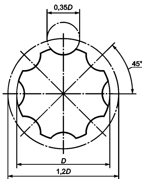
Рисунок 201.102 — Форма рукоятки настройки скорости потока кислорода
